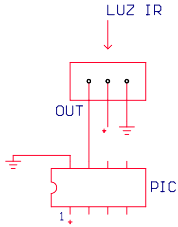
CLAVE 2109 SENSOR IR METALICO
