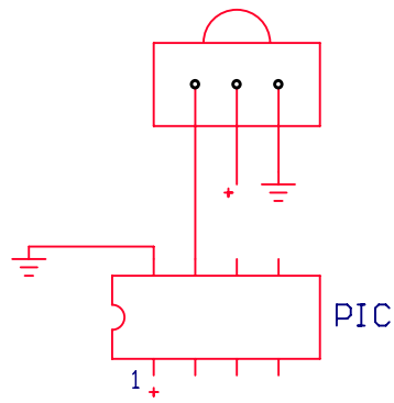
CLAVE 2108 SENSOR IR PLASTICO
